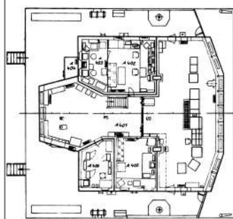
4. Палуба надстроек Aufbaudeck
