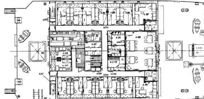
2. Палуба надстроек Aufbaudeck
