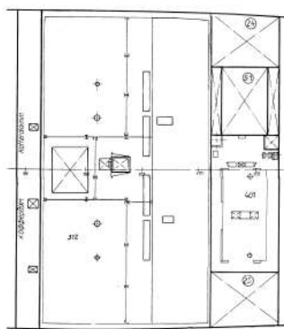
Сечение под 1-й твиндеком Schnitt unter 1. Zwischendeck
