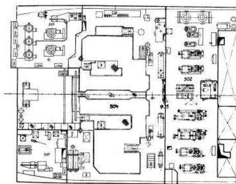
Сечение под 1-й твиндеком Schnitt unter 1. Zwischendeck
