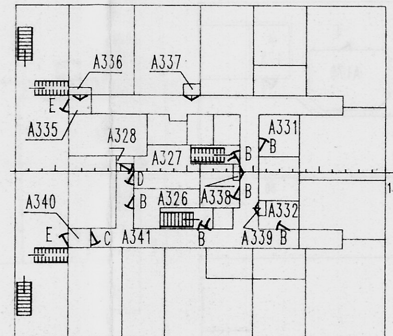
3. AUFBAUDECK 3-Я ПАЛУБА НАДСТРОЕК
