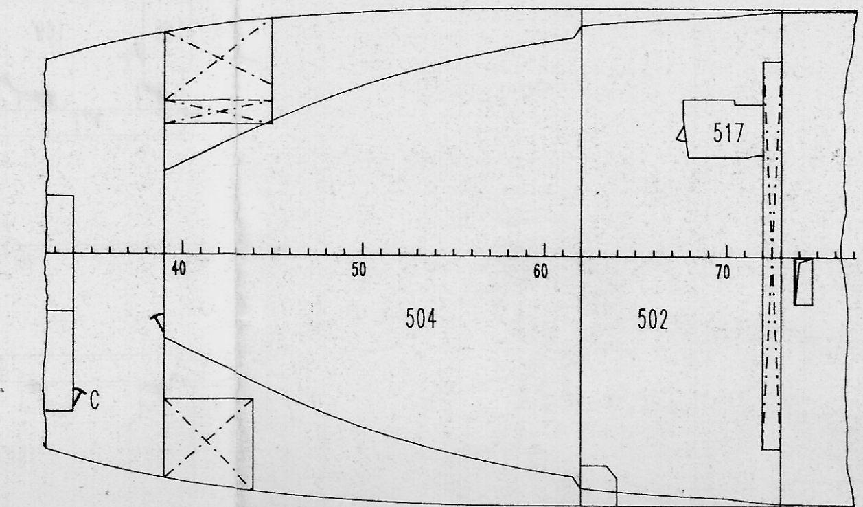
SNITT UEBER STAUNUNG СЕЧЕНИЕ НАД ДВОЙНЫМ ДНИЩЕМ
