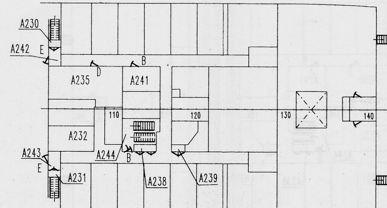
2. AUFBAUDECK 2-Я ПАЛУБА НАСТРОЕК
