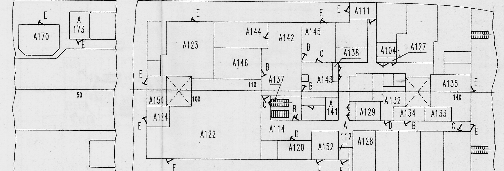
1. AUFBAUDECK 1-Я ПАЛУБА НАСТРОЕК
