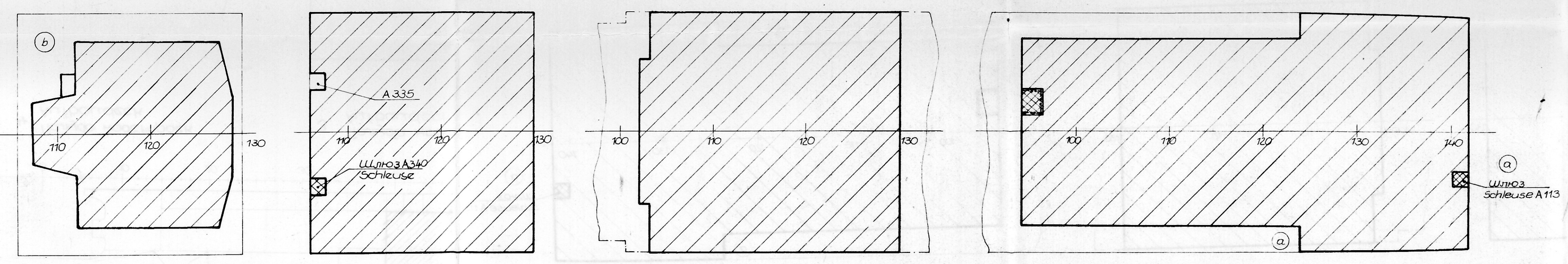
4. Палуба надстроек Aufbaudeck 3. Палуба надстроек Aufbaudeck 2. Палуба надстроек Aufbaudeck 1. Палуба надстроек Aufbaudeck
